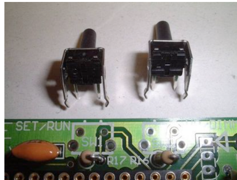
Abbildung 18: Die Taster – zum Stellen der Uhr
