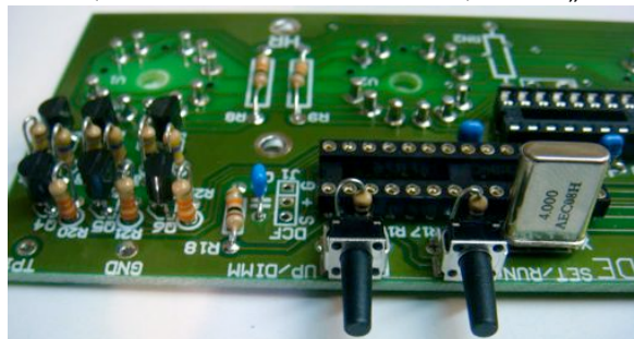
Abbildung 12: Taster, Quarz, Transistoren
