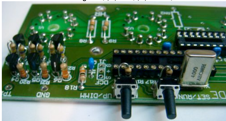
Abbildung 14: Transistoren in Platine
