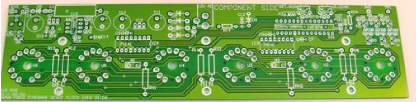
Abbildung 1: Die Komponentenseite der Platine
