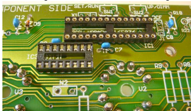
Abbildung 7: die Sockel für die ICs, Kondensatoren
