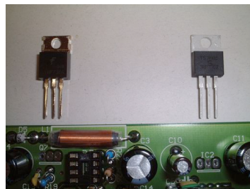
Abbildung 19: Q7 (FET) und IC 2 (7805)
