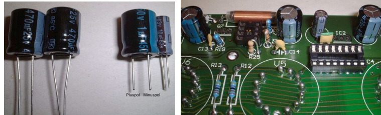
Abbildung 16: Kondensatoren C3, C4, C11, C10
