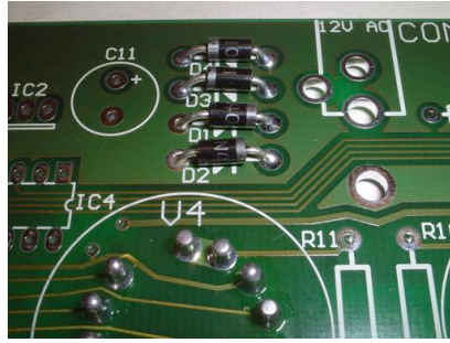
Abbildung 5: Dioden eingelötet und Ansicht der Bestückungsseite der Platine
