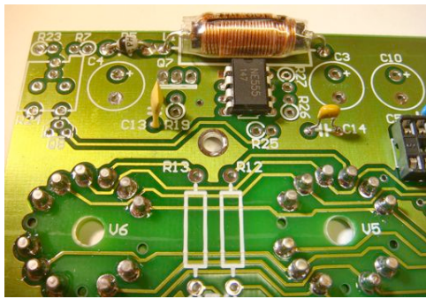
Abbildung 8: NE-555 wird ohne Sockel eingelötet
