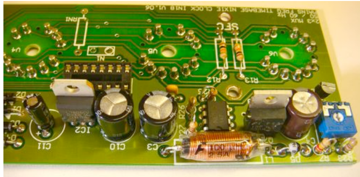
Abbildung 10. die Spule, Kondensatoren, IRF730, 7805, NE-555, Diode D6, Trimmer
