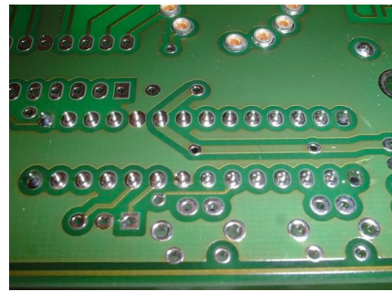
Abbildung 9: 4 Pins außen verlötet.
